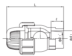
SOCKET END
