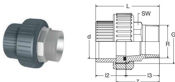
BR PVC-U-GJMW/EPDM Ü-Verschraubung AG-keg grau
