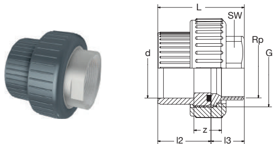
BR PVC-U-GJMW/EPDM Ü-Verschraubung IG-zyl grau
